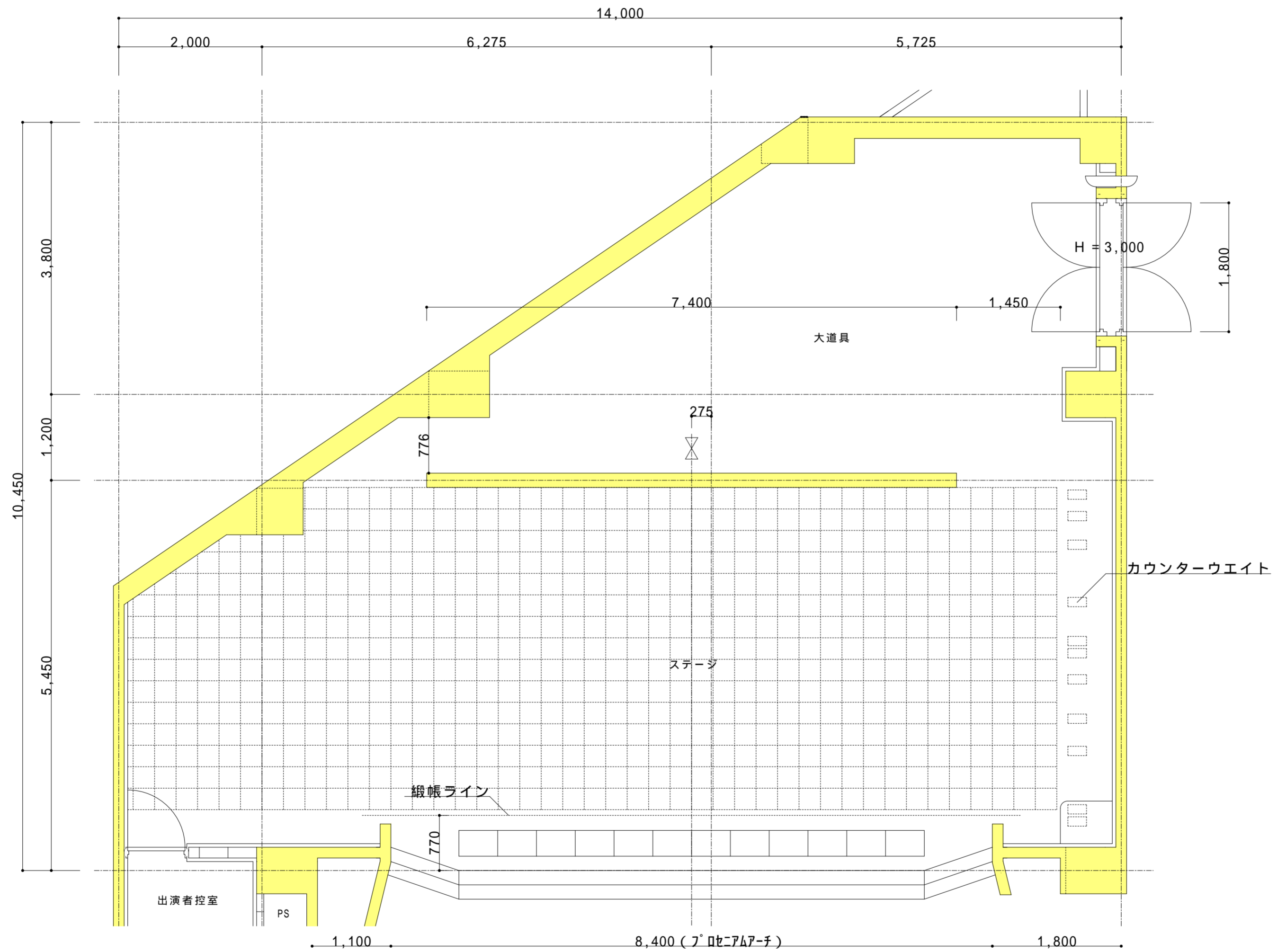
舞台平面図 (白図) マス目30cm角
